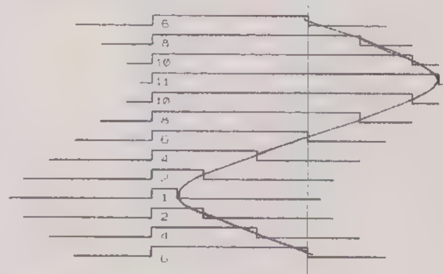
Fig.5 Puls breedte modulatie (PWM).
